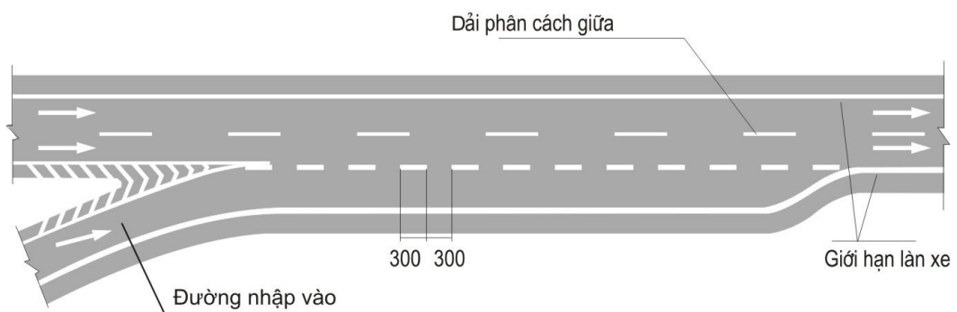
Hình G.20 -Vạch số 18: Vạch nhập làn có đoạn chuyển tiếp kiểu song song.
