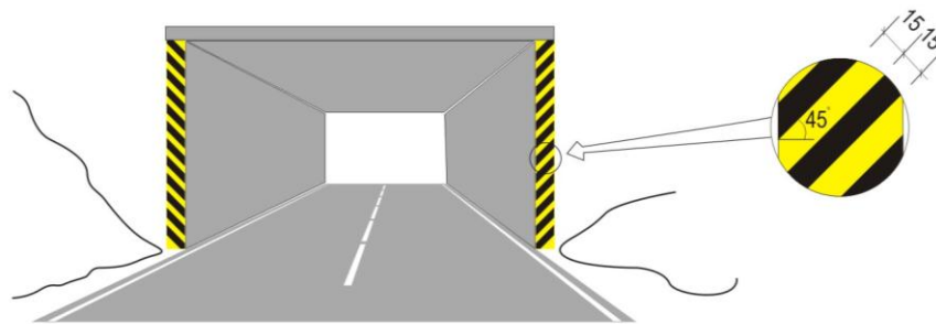
Hình G.75 – Vạch số 68: Tiêu mốc đứng, đơn vị: cm
