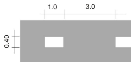
Hình H.8 – Vạch số 1.8, đơn vị m
