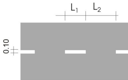
Hình H.5 – Vạch số 1.5, đơn vị m
