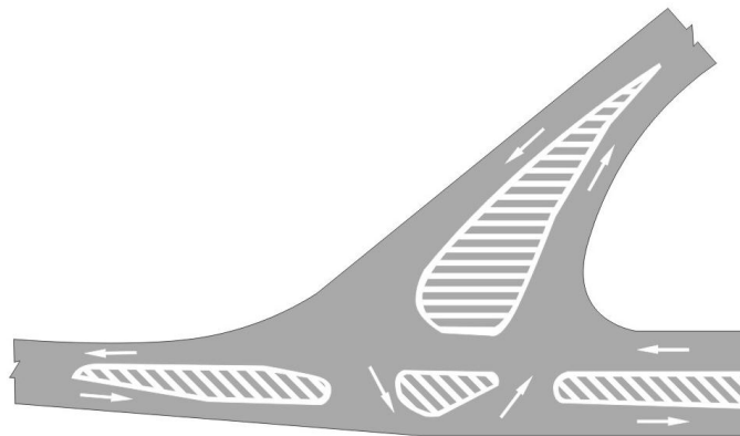
Hình G.53 – Vạch số 46: Vạch phân làn xe ở ngã ba phức tạp
