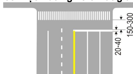
Hình G.46 – Vạch số 39: Kích thước của vạch dừng xe, đơn vị cm.
