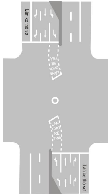
Hình G.7 -Vạch số 7: Vạch làn chờ rẽ trái, đơn vị cm
