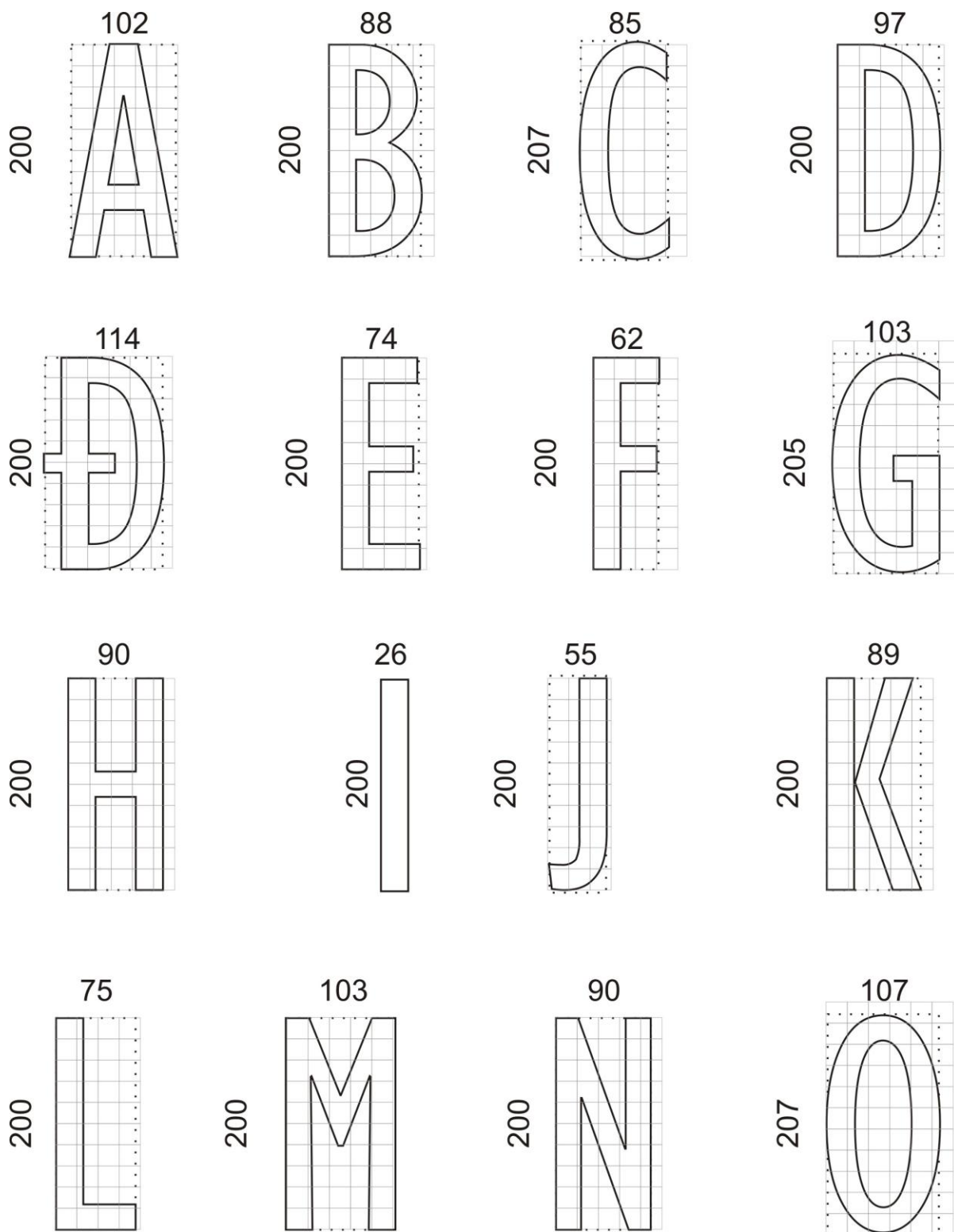
Hình K.3 – Chi tiết chữ viết và con số nét gầy, đơn vị mm
