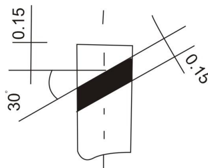
Hình H.27 – Vạch số 2.4, đơn vị m
