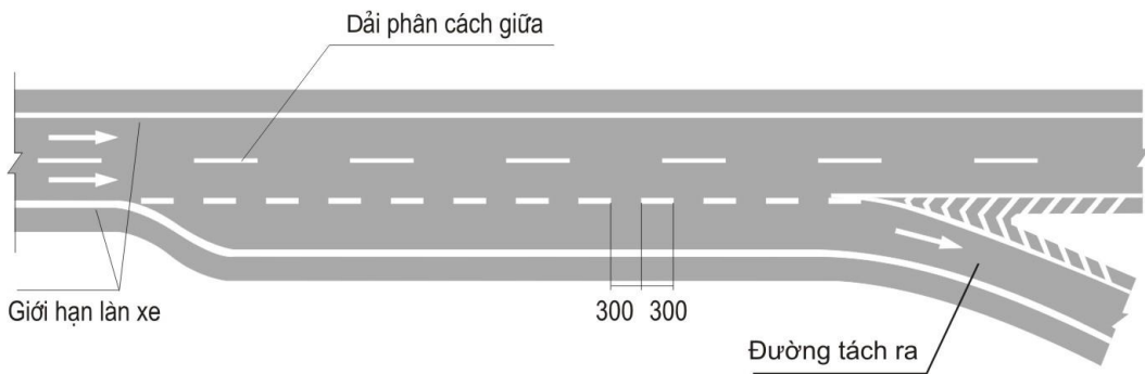
Hình G.17 -Vạch số 15: Vạch tách làn kiểu trực tiếp, đơn vị cm.
