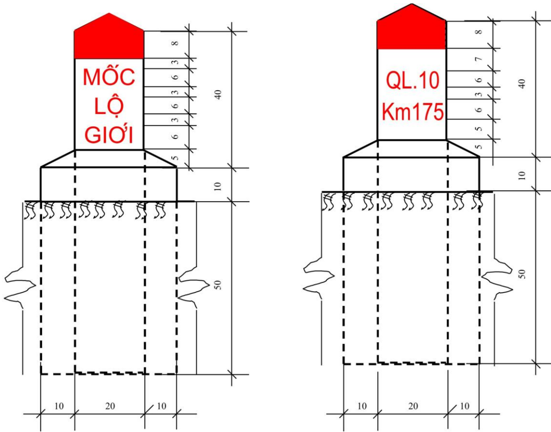
a) Mặt chính (nhìn ra phía đường) b) Hai mặt bên (hướng xe chạy)
